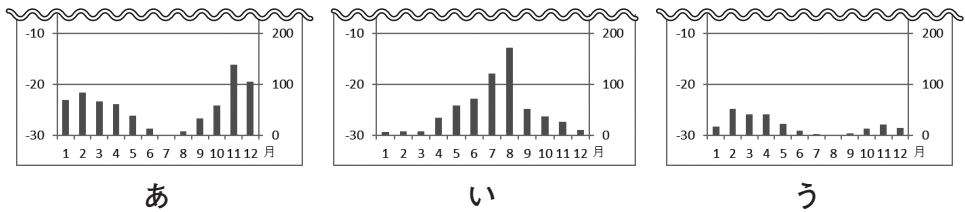
図3 A～Cの月降水量（雨温図下部）
