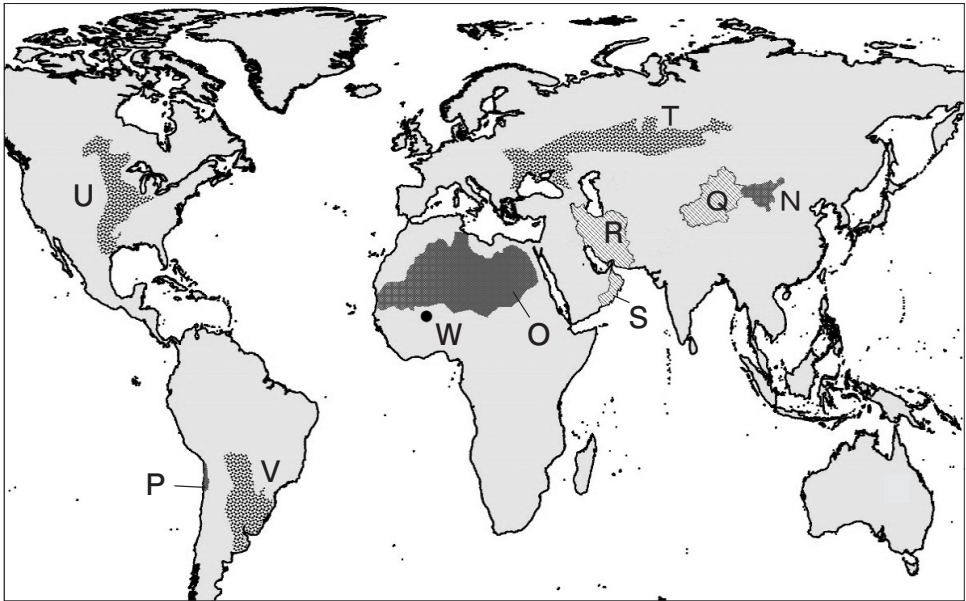
図4 世界の乾燥・半乾燥地域
