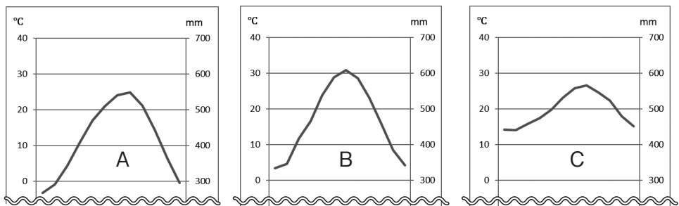
図2 A～Cの月平均気温（雨温図上部）
