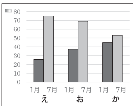
図6 1月と7月の降水量
