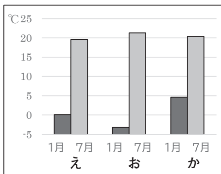
図5 1月と7月の気温
