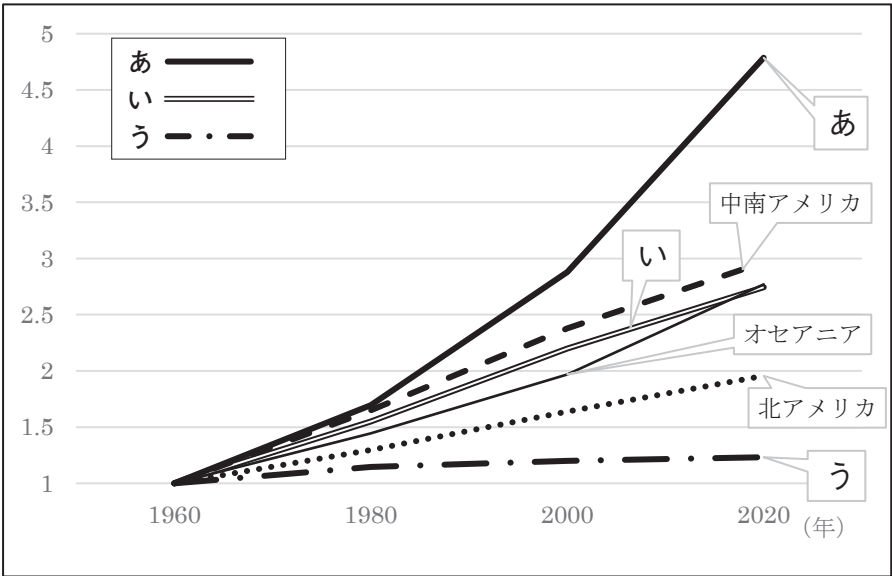
図1 世界の人口推移
