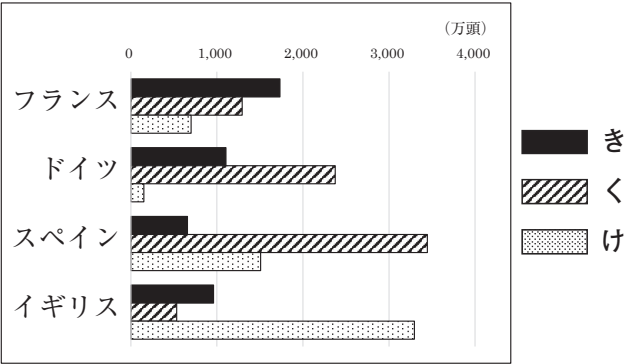
図 10 主な国の家畜飼育頭数 (2021 年)
